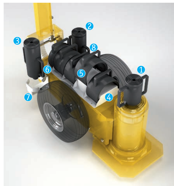
A05102 Safety device system - Kit blocchi di sicurezza
